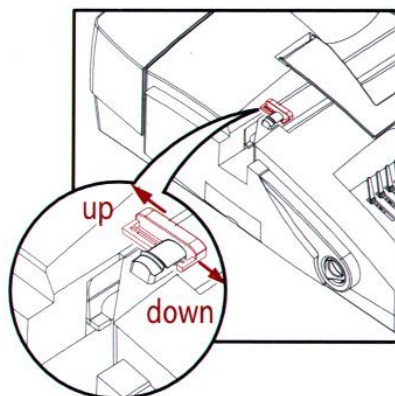
Obrázek – 2. (výběr děrovací štěrby) Posuňte vodítko děrovací štěrby (5) (část červené oblasti) nahoru pro děrování dírek A4, LTR (dopisní), US – americké rozteče. Posuňte vodítko děrovací štěrby (5) dolů pro děrování extra velkých papírů (A3 ... atd.).
