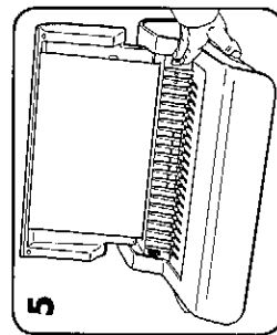
5. Otestujte děrování na nepotřebných listech pro kontrolu nastavení vodítka okraje.
